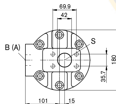
View Y
